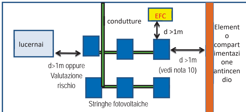
Esempio di distanze minime di EFC, lucernai e elementi di compartimentazione dai componenti dell'impianto fotovoltaico
