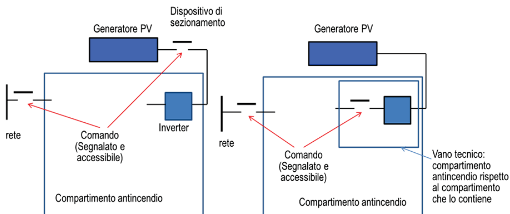
Esempi di possibili modalità di messa in sicurezza
